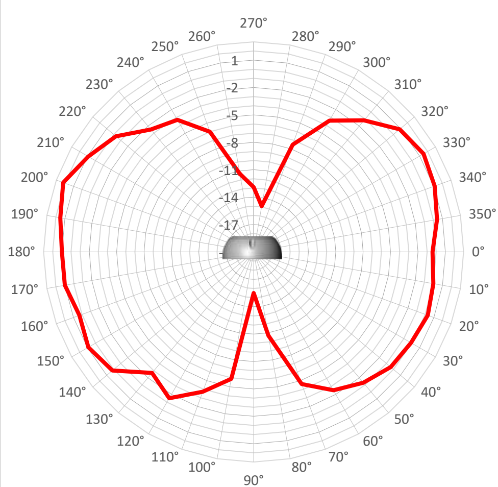
АК 2.7-9 в вертикальной плоскости 2800МГц
