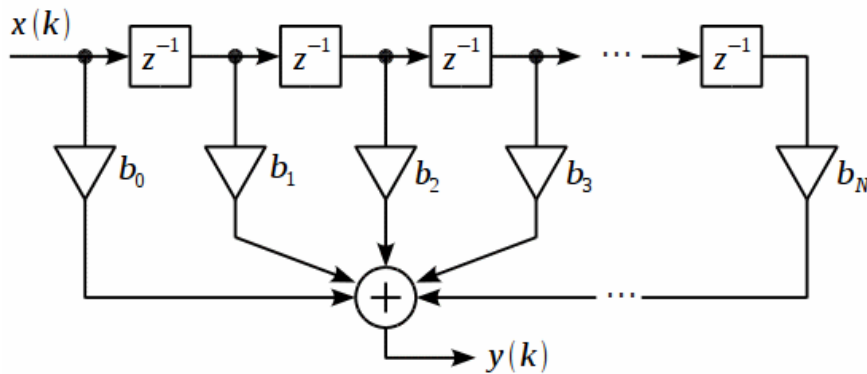
Рис.1 – Структурная схема нерекурсивного КИХ-фильтра
