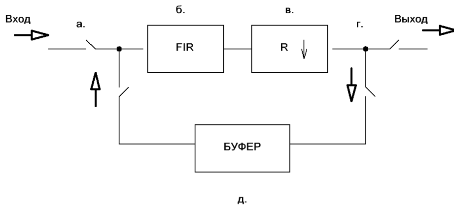
Рис.1. – Структурная схема буферного КИХ фильтра:
