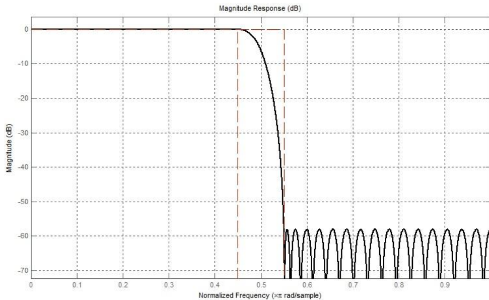
Рис.4а.– АЧХ КИХ фильтра ( n = 62 , w_{pass} = 0.45 , w_{stop} = 0.55 ).
