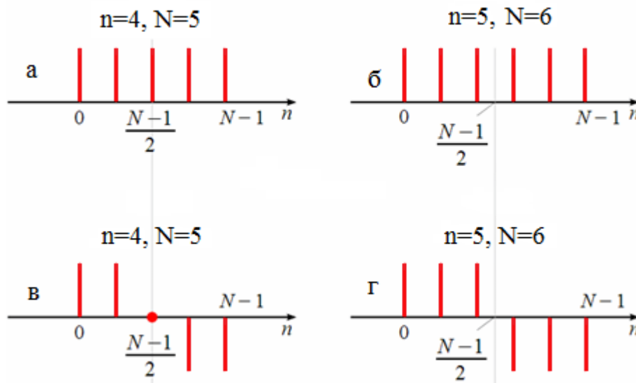
Рис.3 – Типы импульсных характеристик КИХ фильтров
