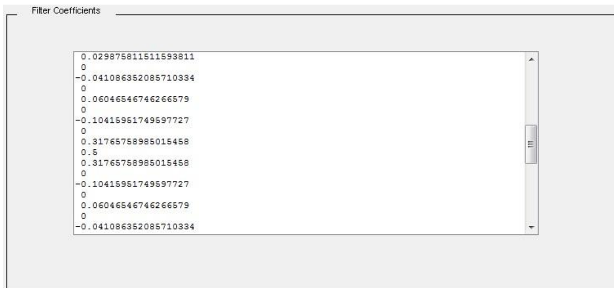
Рис.4б. – Коэффициенты КИХ фильтра (n=62, wpass 0.45, wstop = 0.55).
